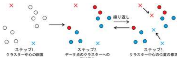
図 1 k-means 法
